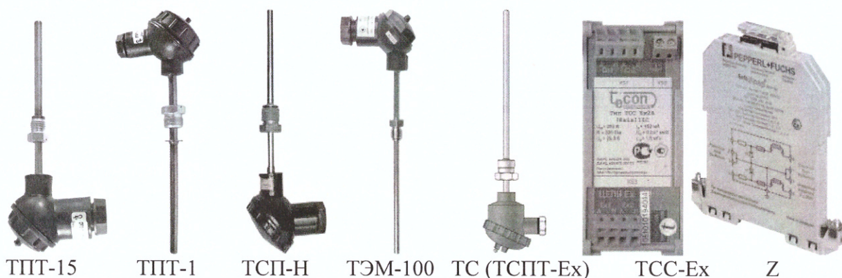
Рисунок 5 - Преобразователи температуры
