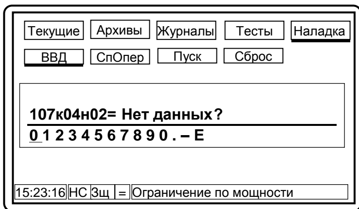
Рисунок 5.19 – Пример набора номера параметра, канала и индекса
