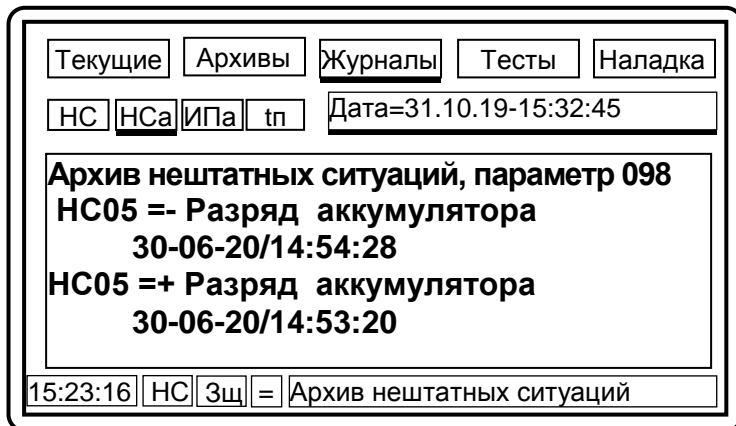
Рисунок 5.8 – Вывод на дисплей информации из архива НСа
