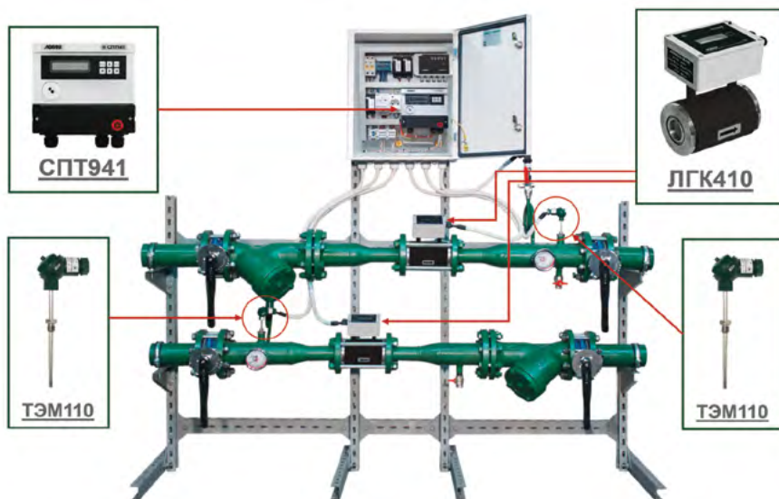
ЛГК410 в составе узла учета тепловой энергии
