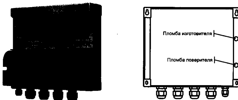
Рисунок 1 – Общий вид и схема пломбирования (вид сзади)
